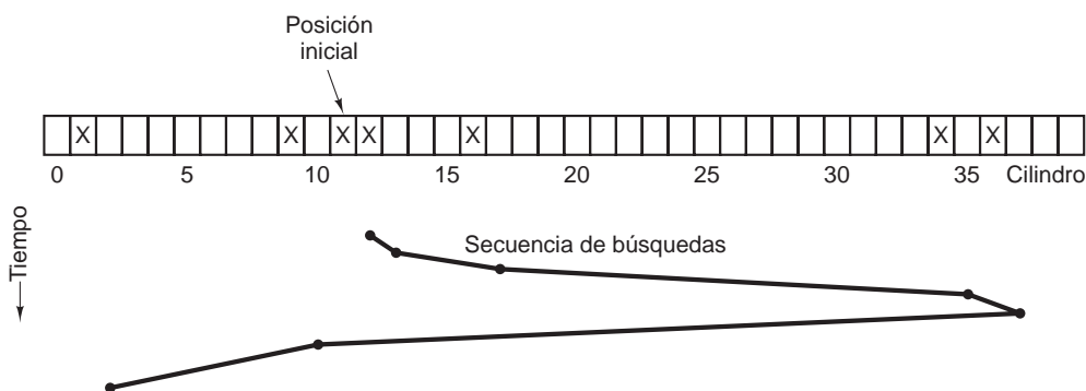
Figura 5-29. El algoritmo del elevador para planificar las peticiones de disco.
