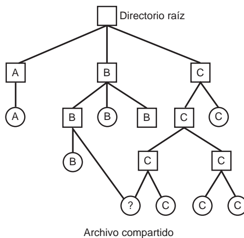
Figura 4-16. Sistema de archivos que contiene un archivo compartido.
