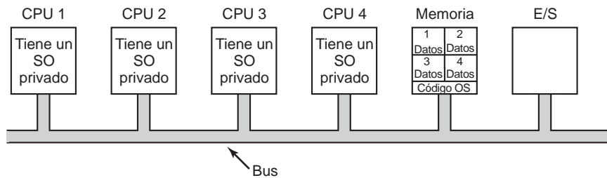
Figura 8-7. Particionamiento de la memoria de un multiprocesador entre cuatro CPUs, pero compartiendo una sola copia del código del sistema operativo. Los cuadros marcados como Datos son los datos privados del sistema operativo para cada CPU.
